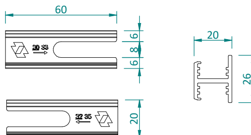
(B) Morsetto finale universale Omni Fix - accessorio di regolazione
