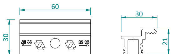
(A) Morsetto finale univiersale OmniFix - componente fisso
